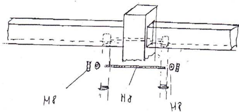
Skizze für die Pfostenmontage beim Brüstungsgeländer der Spindeltreppe "Lugano"
